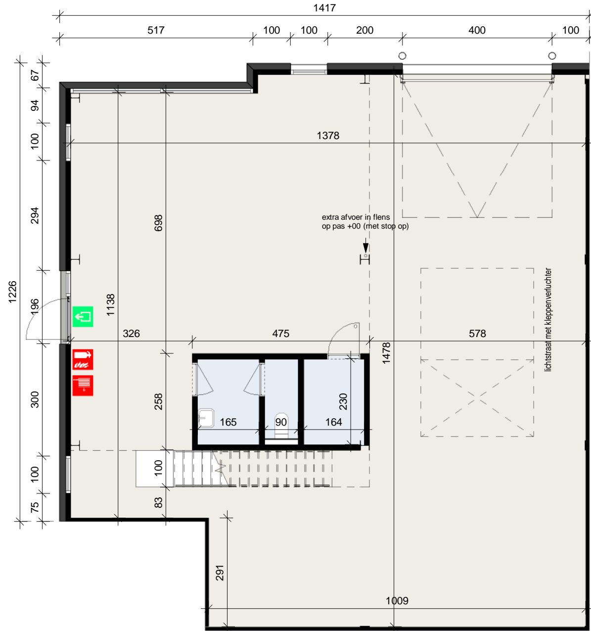
Gelijkvloers
