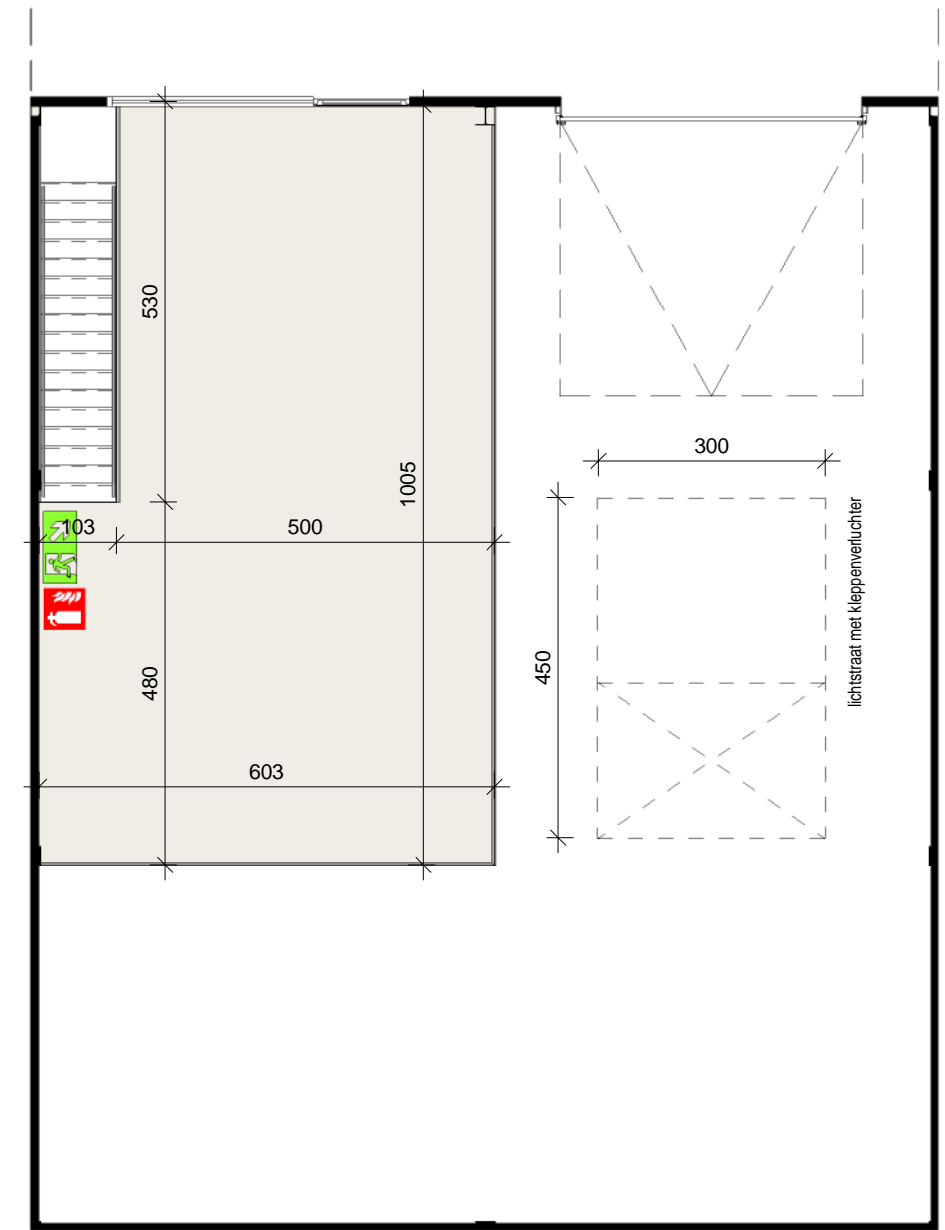
Verdieping 1 1 : 100
