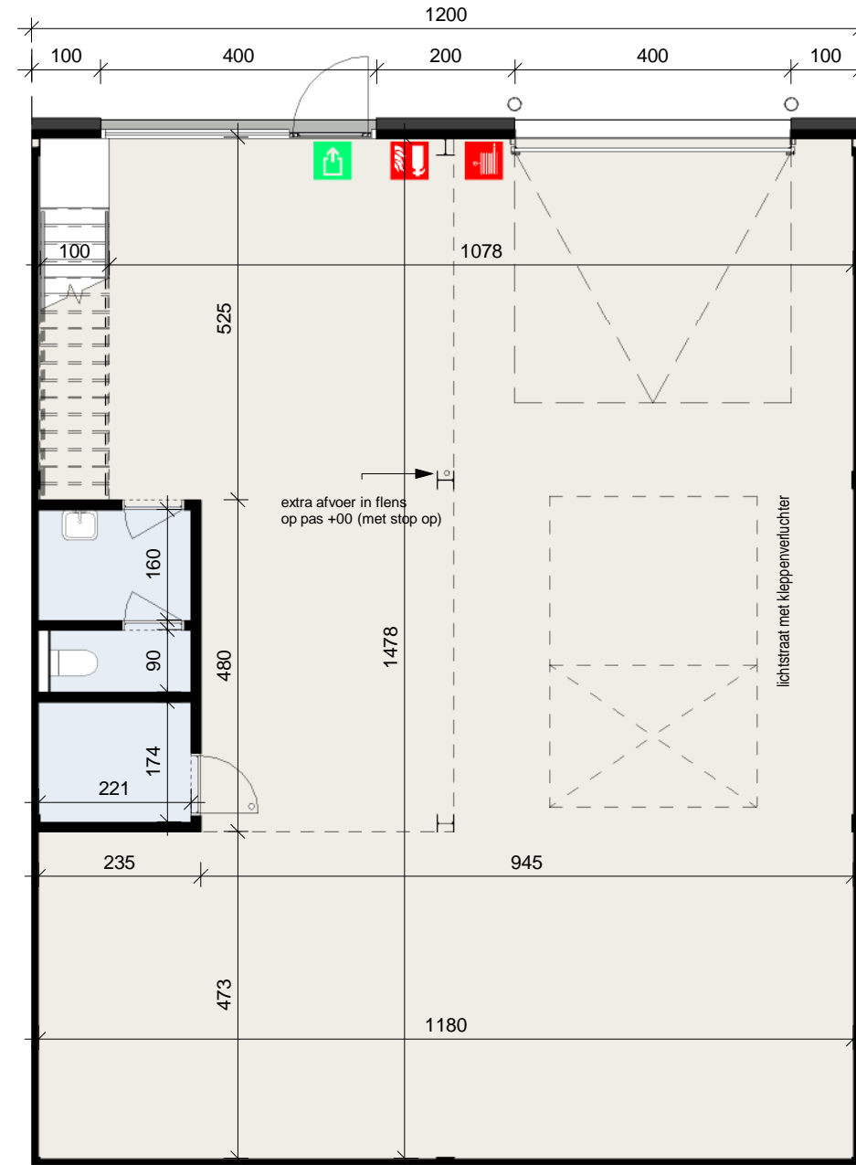
Gelijkvloers 1 : 100
